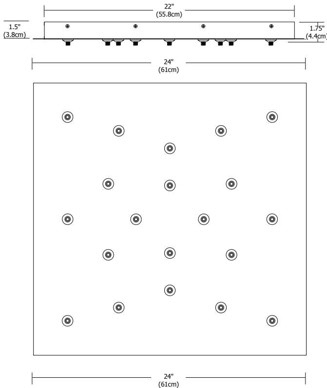
20-Port Canopy
