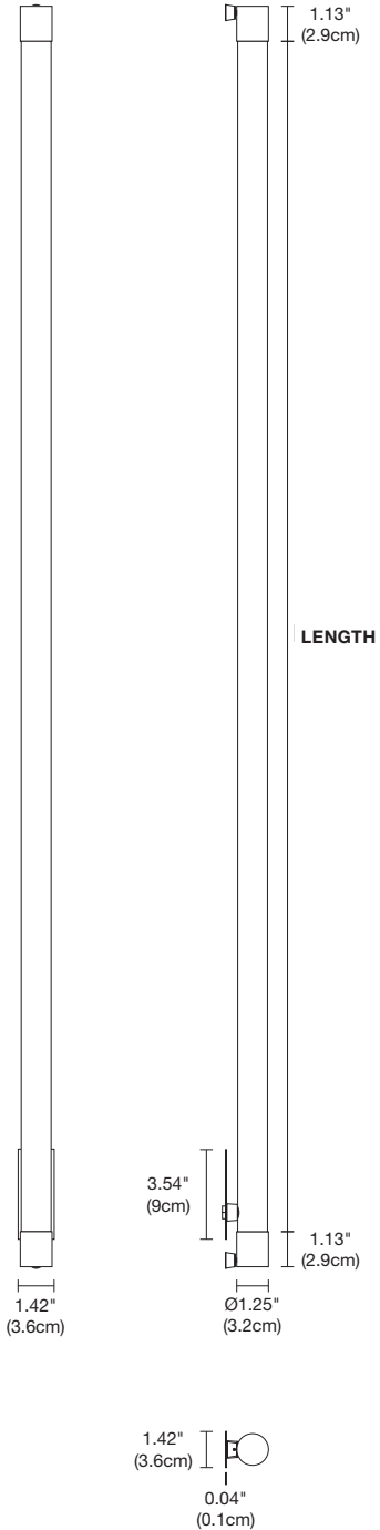
E1R - End Power Feed 1" Rectangle Canopy
